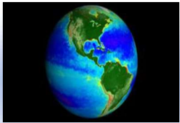
Earth
