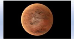
Venus
